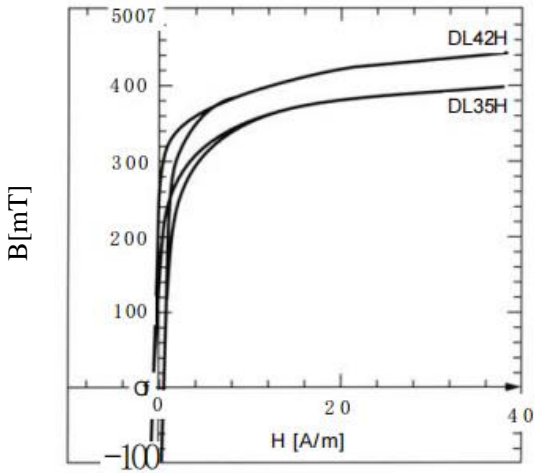
DL42H, DL35H B~H曲线
