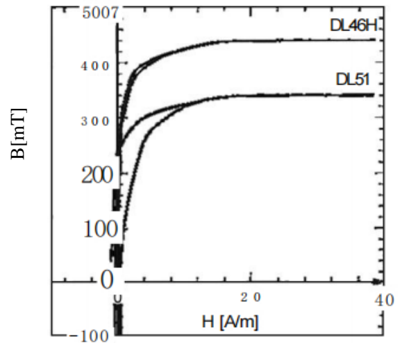
DL46H, DL51 B~H曲线
